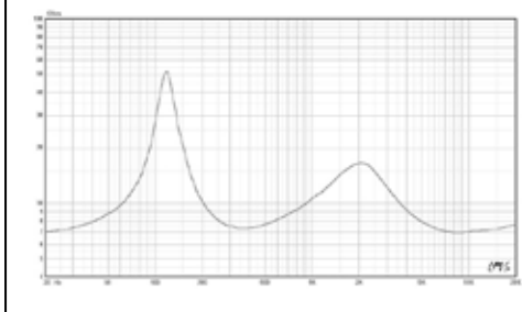
Graphique d'Impédance::
